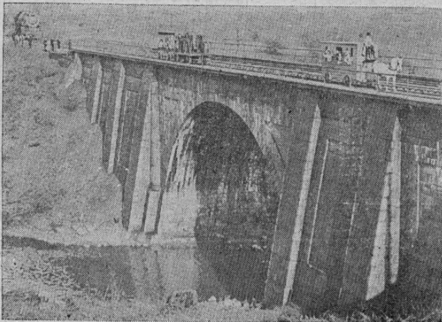
El puente Carrollton, cerca de Baltimore, Maryland, fué construido hace más de cien años, y es el más antiguo en el servicio ferroviario. Tan bien construido está, que todavía lo cruzan los más pesados trenes del sistema Bantimore-Ohio
