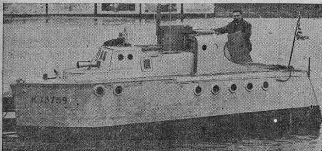
David R. Huber, de Avon, Nueva Jersey, a quien se ve aquí a bordo de su barco, en SILVER DREAM, de 19 pies de largo, de acero reforzado con concreto, espera hacer un viaje al redor del mundo en dicha embarcación.
